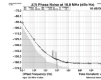
ST 36系列典型测试曲线
