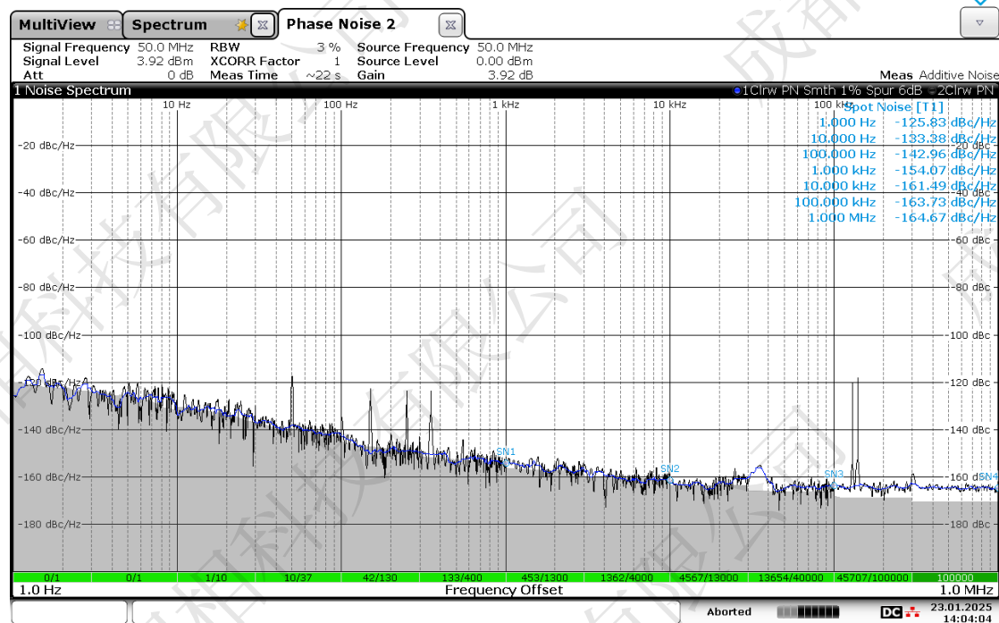
50MHz 相位噪声相噪曲线
