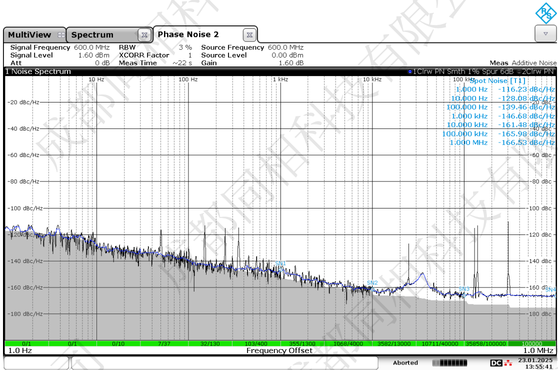
600MHz 相位噪声相噪曲线
