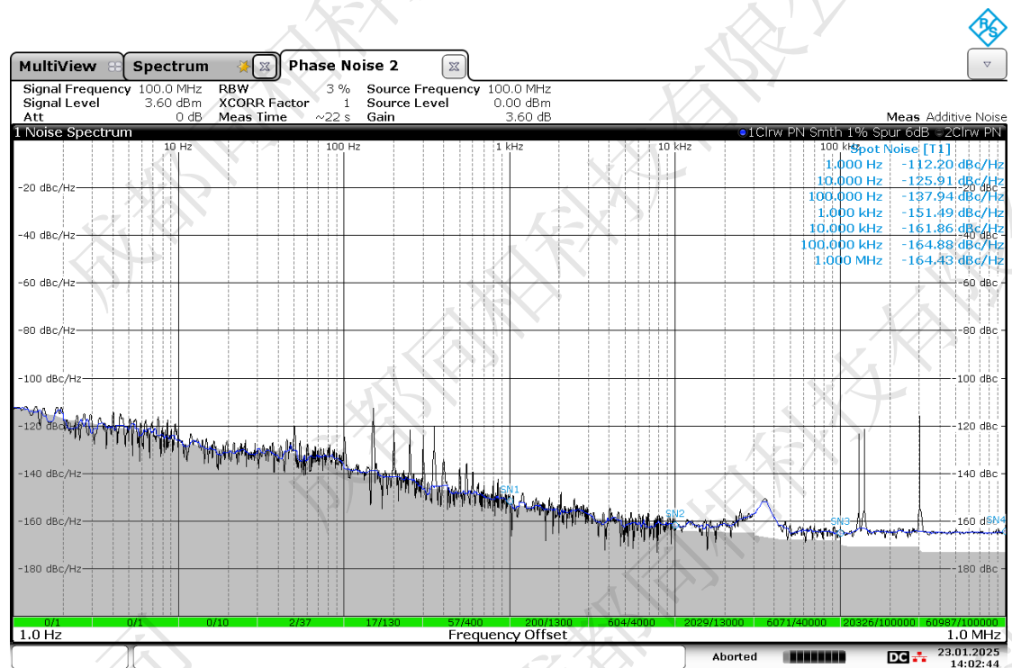
100MHz 相位噪声相噪曲线
